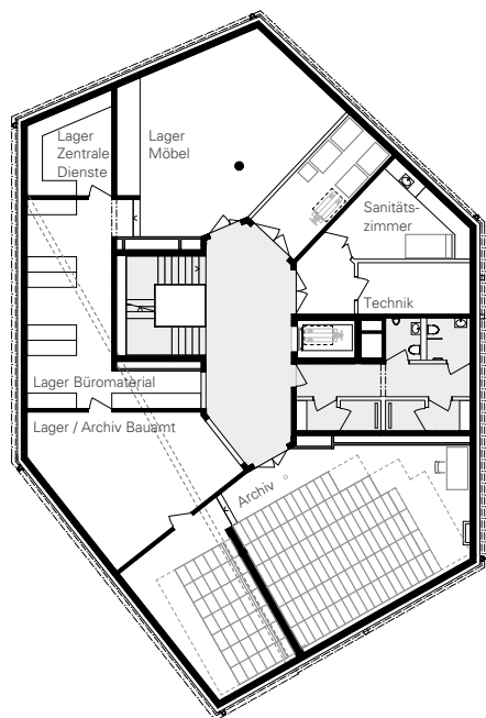
1. Untergeschoss
