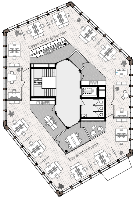
1. Obergeschoss
